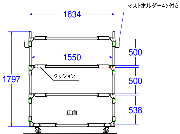
オプションキャスター付図面
