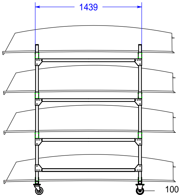
自在キャスター (オプション) 固定キャスター (オプション) 側面
