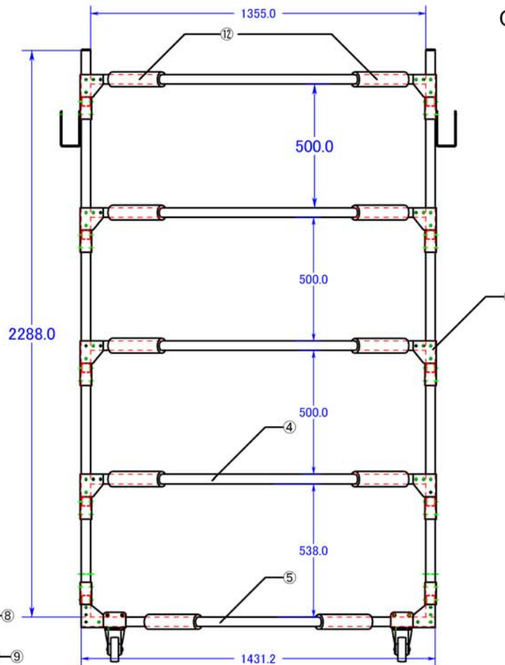
後面図
