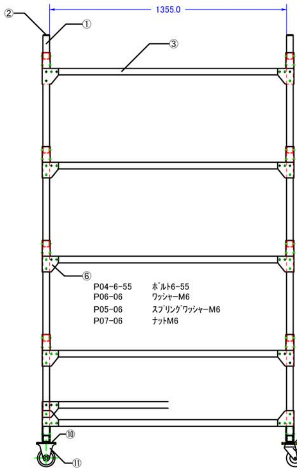
側面図
