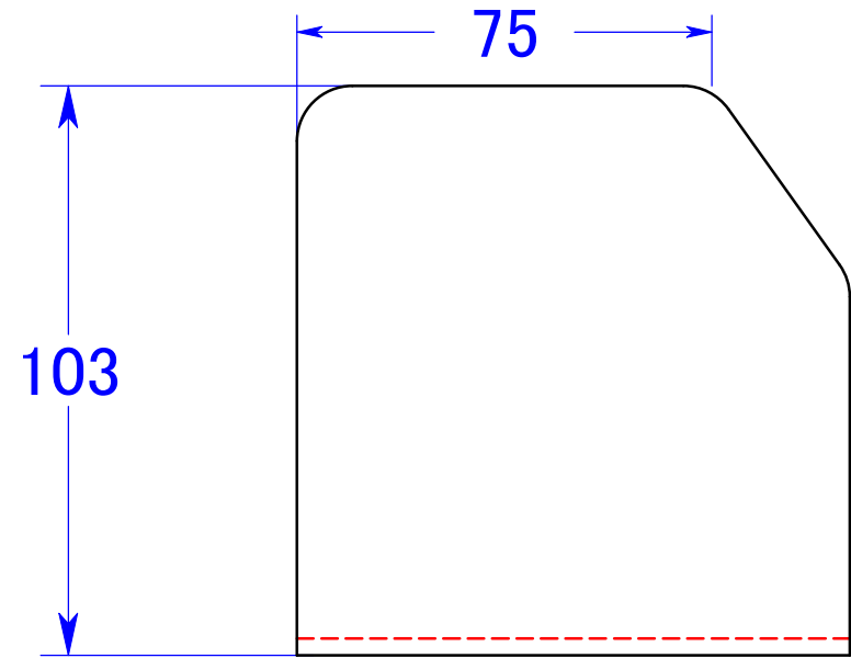
6002 ズブシートリフトベースラケット用大Sバー付（スターボード側）
